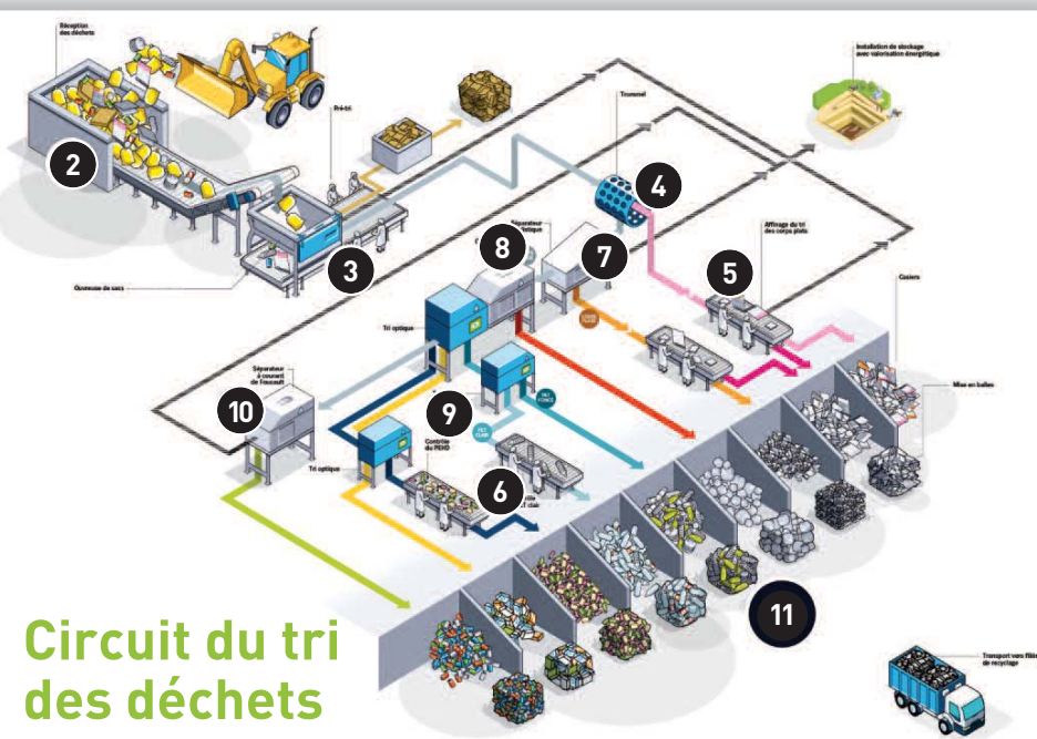
2 Les déchets sont versés dans une trémie de chargement pouvant contenir jusqu'à 6 tonnes de produits. Elle est équipée d'un ouvre-sac qui lacère les sachets afin de libérer les déchets. À la sortie de l'alimenteur, ils sont déposés sur un tapis qui les mène vers la cabine de pré-tri.
